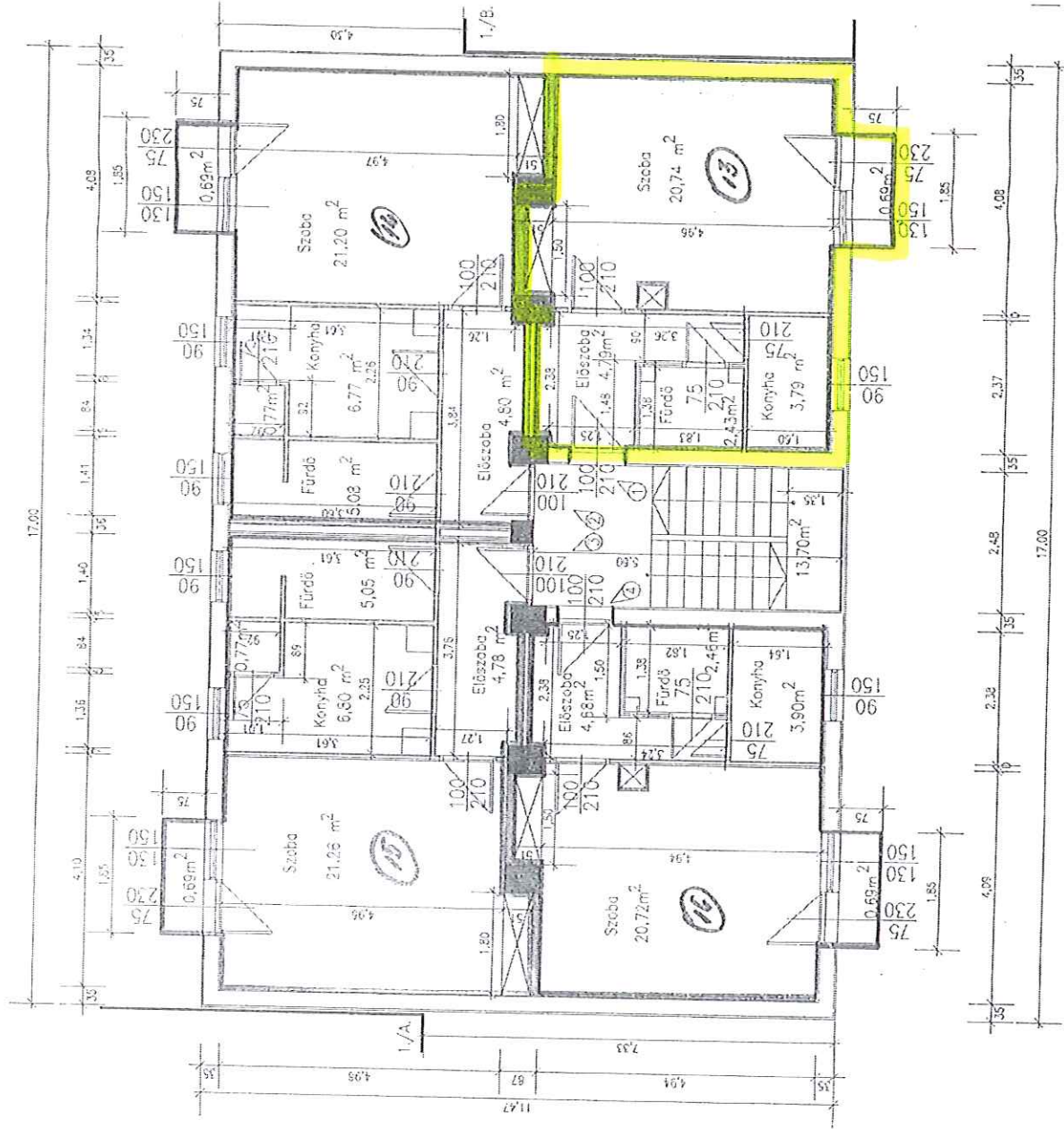
III. EMELETI ALAPRAJZ
